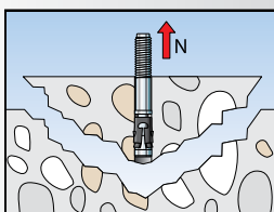
Образование бетонного конуса
